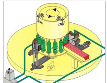
Düsensystem
