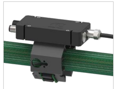
Abgesetztes Elektronikmodul
