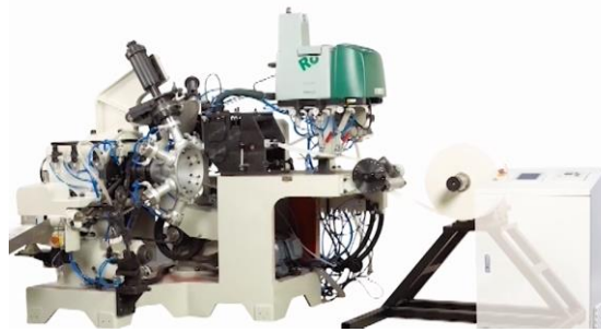
Macchina per coppette di carta di Dayuan con fusore Robatech Concept (in alto) e pistola applicatrice AX Diamond
