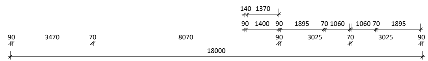
Plan Floor Plan 1 : 100
