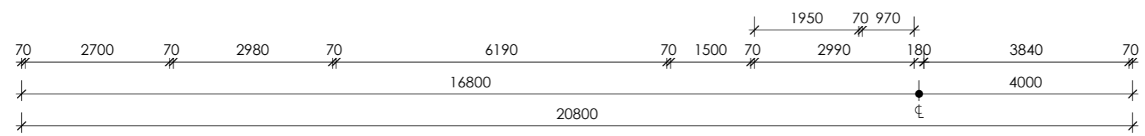
Plan Floor Plan 1 : 100
