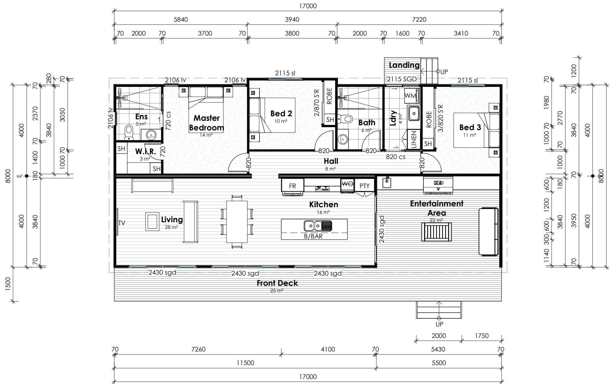
Plan Floor Plan 1 : 100
