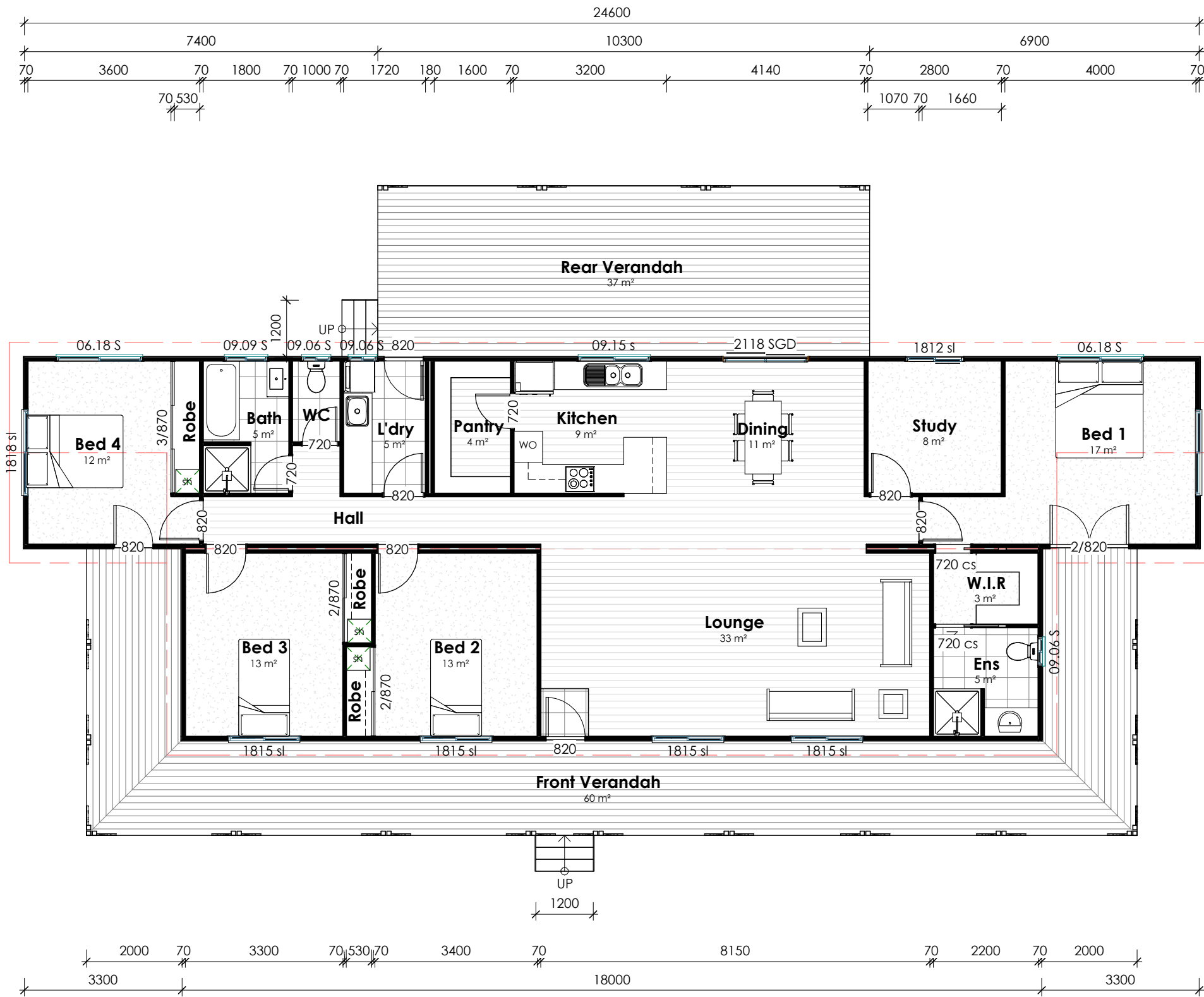
Plan Floor Plan 1 : 100
