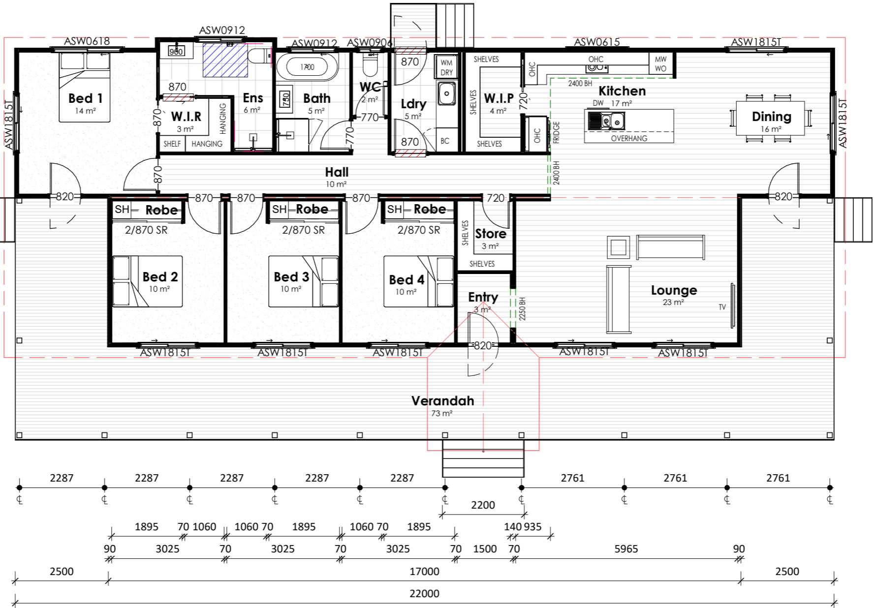
Plan Floor Plan 1 : 100
