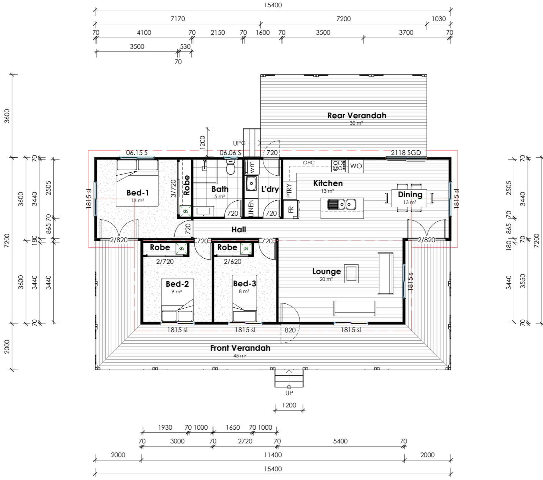
Plan Floor Plan 1 : 100
