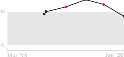
IDEXX SDMA
