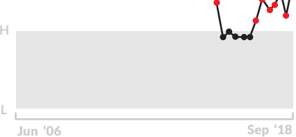
IDEXX SDMA
