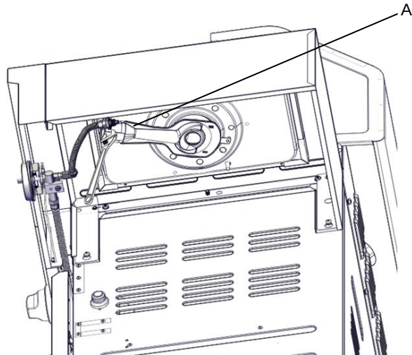
A. Extremo flexible del quemador lateral
