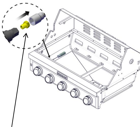
A. Gicleur de brûleur principal
