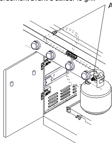
A. Ensemble détendeur/tuyau
