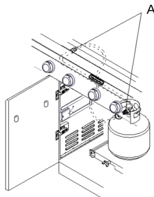
A. Ensamblaje de regulador de presión/manguera de gas
