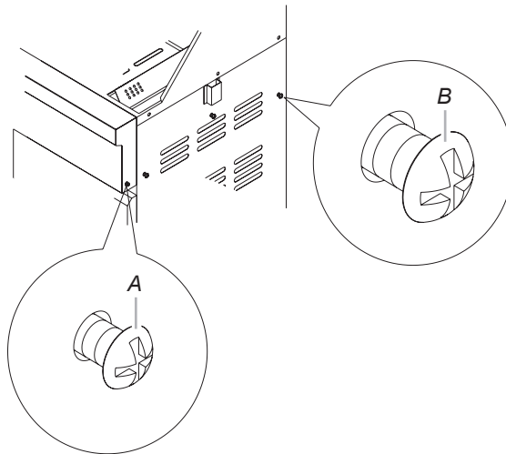
A. Vis du tableau de commande du grill B. Vis du panneau latéral du grill
