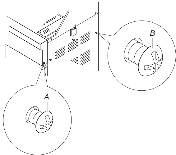
A. Tornillo del panel de control del asador
