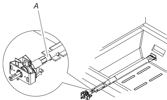
A. Conexión del quemador/orificio
