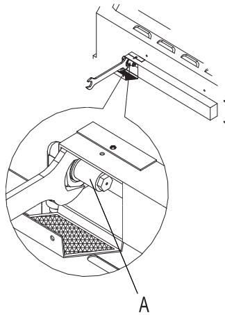
A. Écrou pour gicleur
