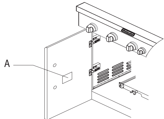
A. Placa con el número de modelo/serie
