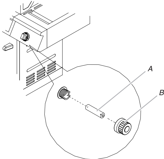
A. Batería de tamaño "AA" B. Tapa del encendedor
