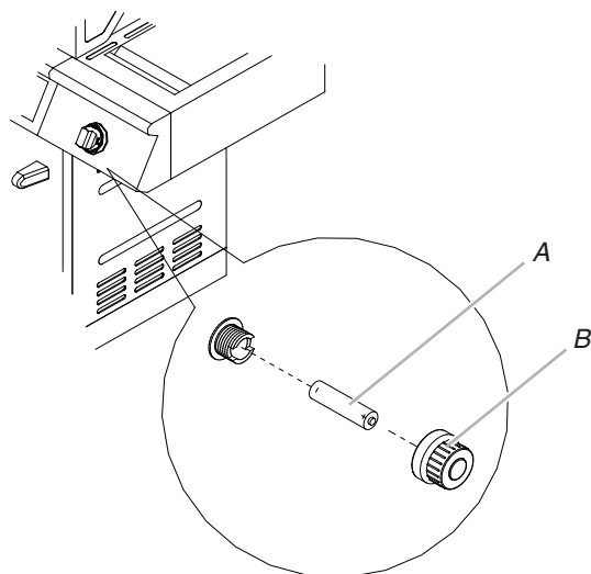
A. Pile de format "AA" B. Couvercle d'allumeur
