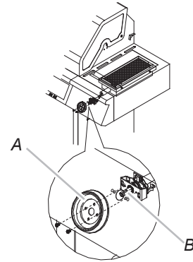
A. Cerclage B. Tige de réglage
