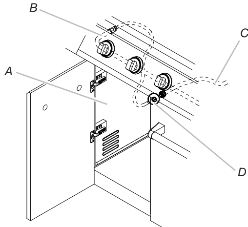
A. Panneau de gauche B. Tubulure de distribution C. Conduit de gaz en PVC de 10 pi (3,0 m) D. Ensemble détendeur/tuyau pour gaz naturel
