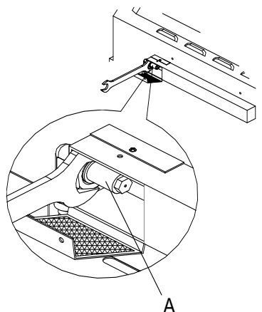
A. Écrou pour gicleur
