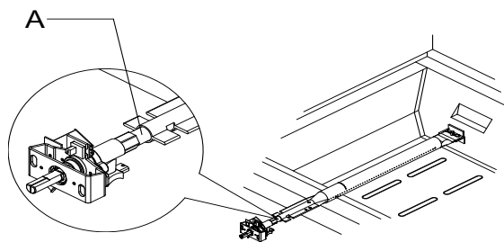
A. Raccordement brûleur/gicleur
