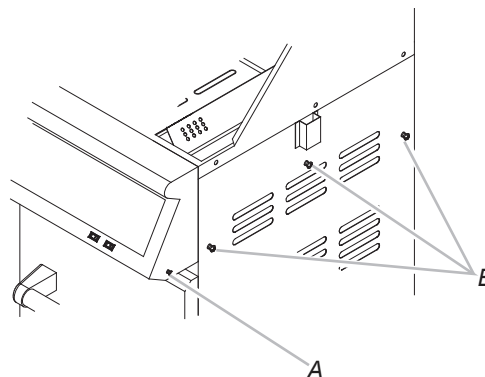
A. Tornillo del panel de control del asador B. Tornillos del panel lateral del asador
