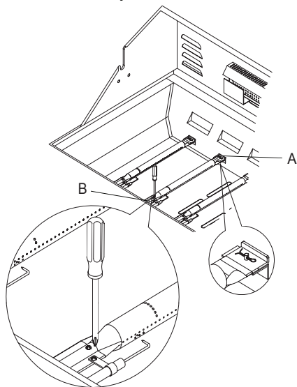
A. Clip B. Tornillo
