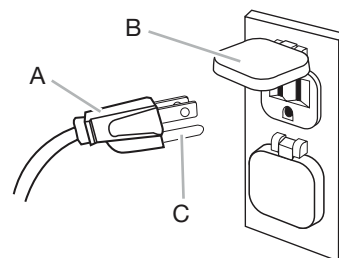
A. Prise à 3 broches reliée à la terre B. Prise d'extérieur polarisée à 3 alvéoles reliée à la terre et à disjoncteur différentiel C. Broche de liaison à la terre
