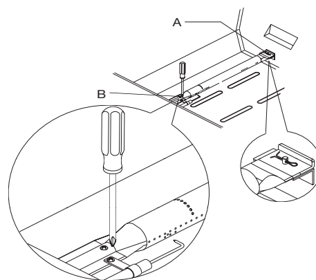
A. Clip B. Screw
