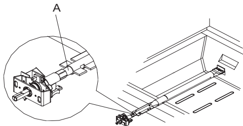
A. Conexión del quemador/orificio
