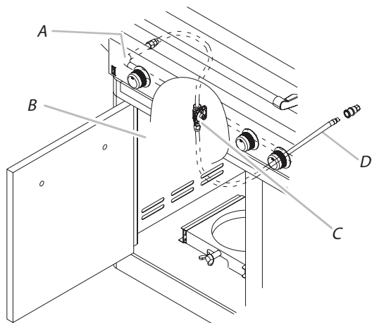
A. Distribuidor B. Panel lateral izquierdo C. Ensamblaje de regulador de presión/manguera de gas natural D. Manguera de gas en PVC de 10 pies (3,0 m)
