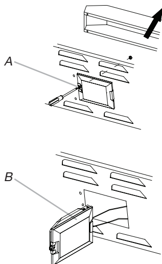
A. Screw B. Light assembly
