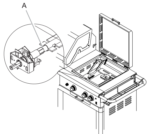
A. Conexión del quemador/orificio
