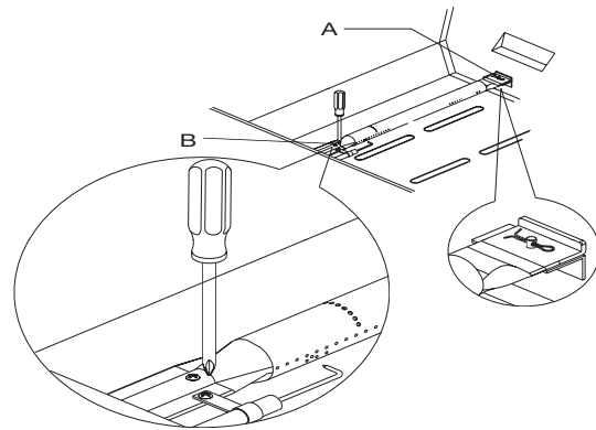
A. Clip B. Tornillo
