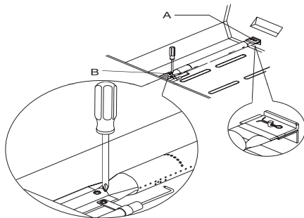
A. Agrafe B. Vis
