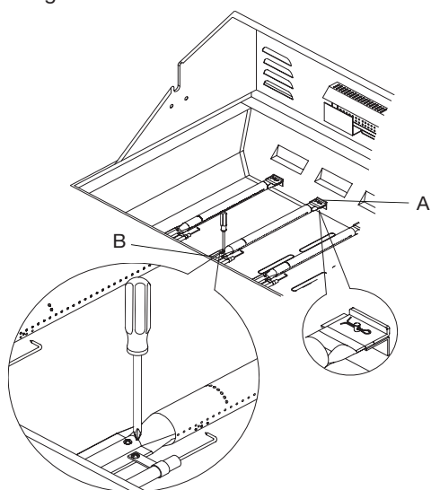
A. Clip B. Screw
