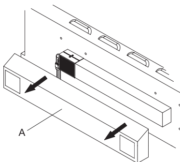
A. Couvercle d'accès
