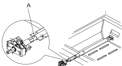
A. Raccordement brûleur/gicleur
