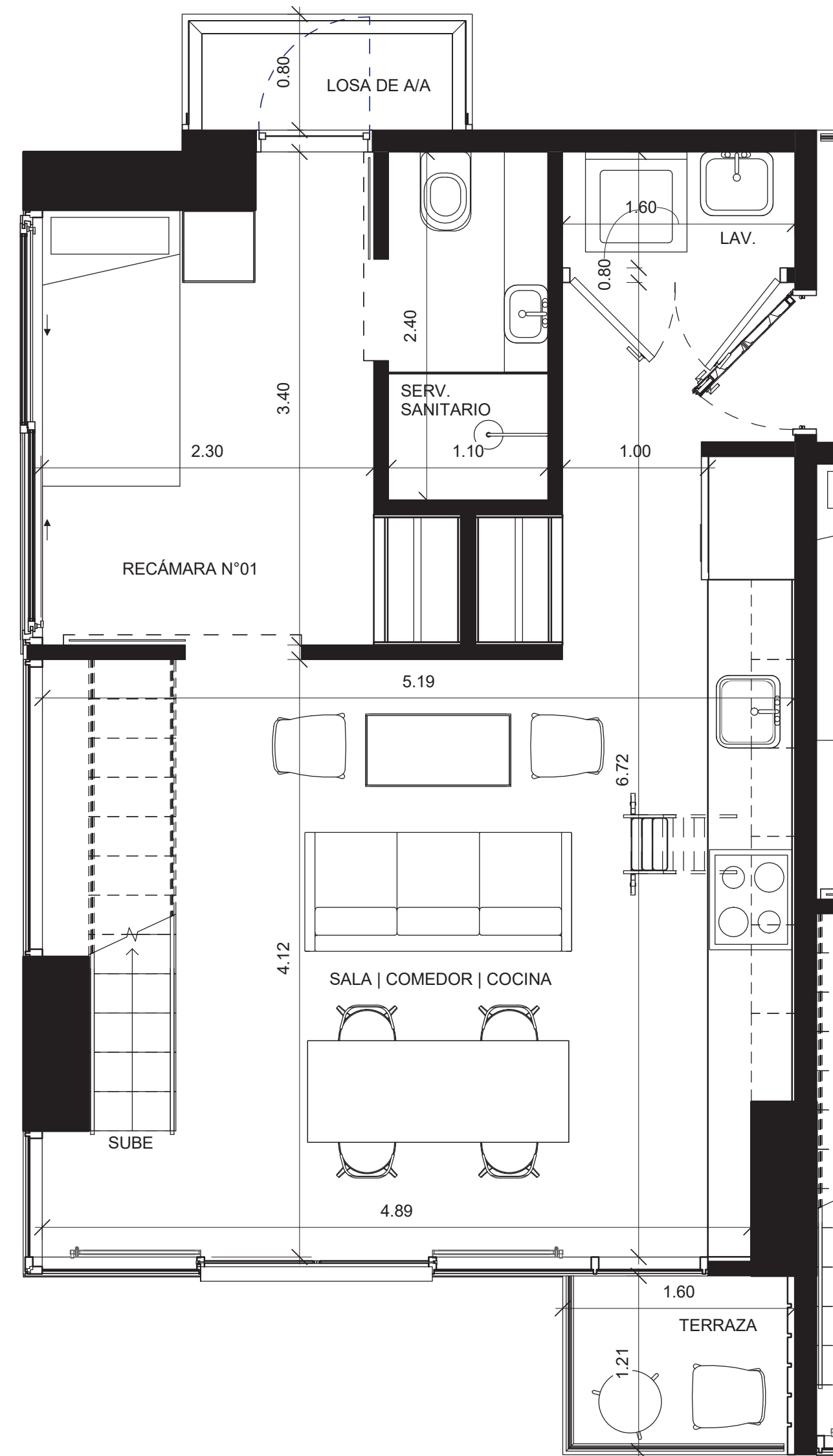
PLANTA BAJA
