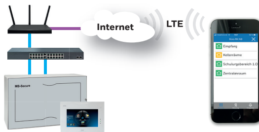
Verbindung mit fester IP über Internet
