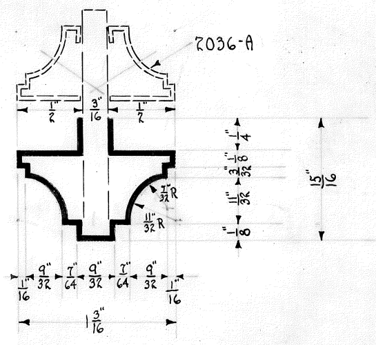
MUNTIN MOULD FOR 1\frac{3}{4} DOOR
